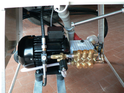
Unité haute pression pour 140 bar
